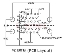
PCB布局 (PCB Layout)
