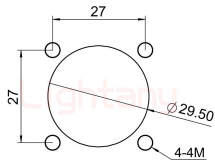
开孔尺寸
